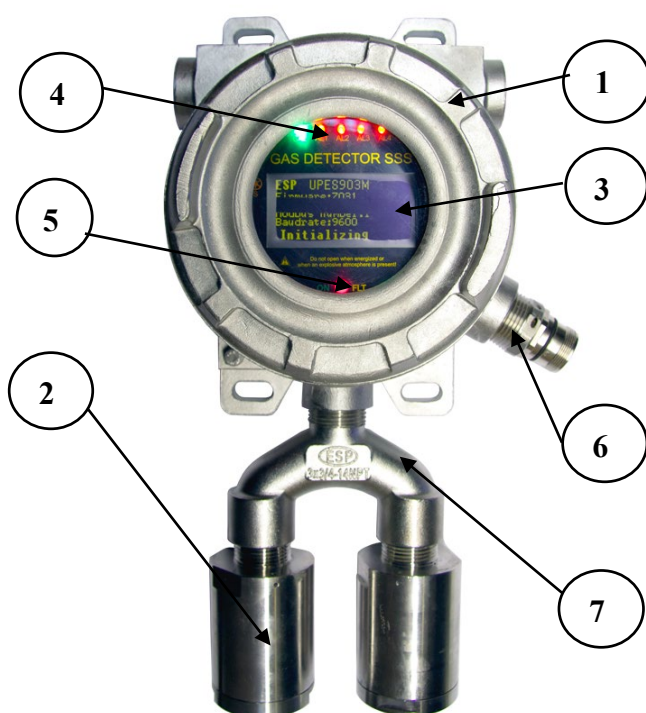
Рисунок 1 - Общий вид газоанализатора CCC-903MT с подключением 2-х преобразователей ПГУ к трансмиттеру ССС (опция «выносного сенсора» ПГУ)
