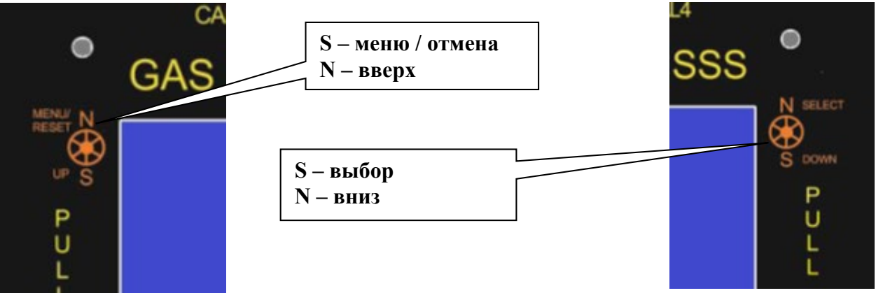
Фальшь панель газоанализатора ССС-903МТ
