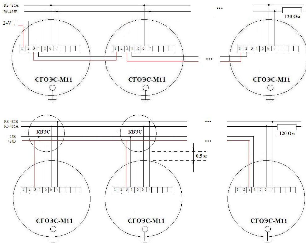
Рисунок 6 – Схемы подключения СГОЭС-М11 в шлейф сигнализации по RS-485
