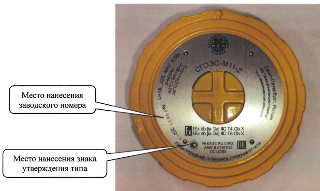
Рисунок 5 – Табличка, расположенная на крышке корпуса газоанализаторов
