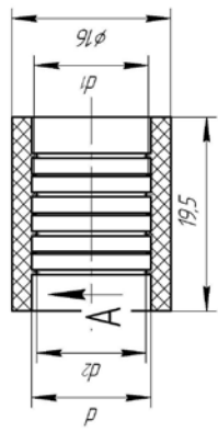
Размеры, мм
